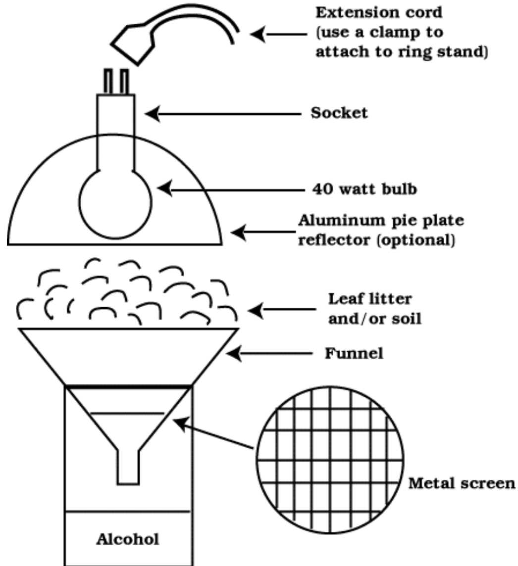
Berlese Apparatus
